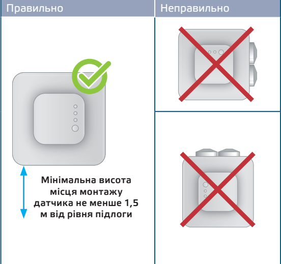
Мал. 5 Монтажне положення
