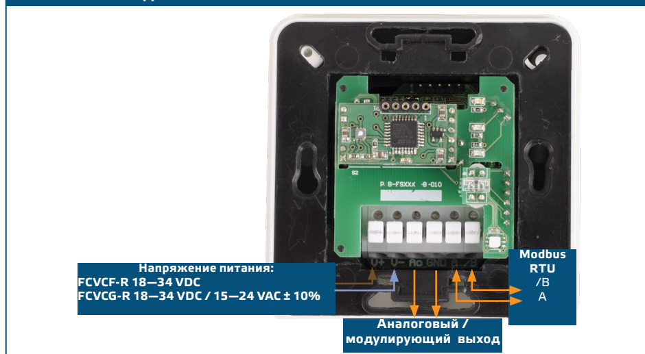
Рис. 1 Схема подключения
