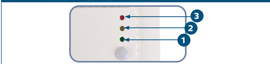
Рис. 6 Светодиодная индикация
