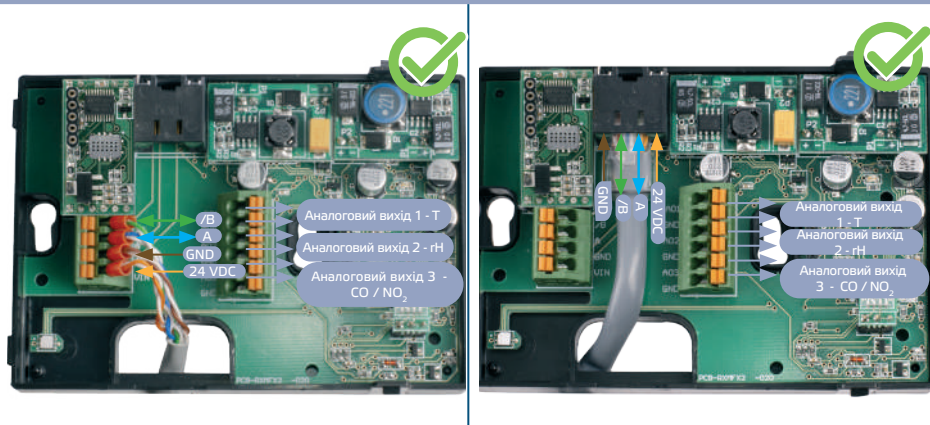
Мал. 4 Схема підключення
