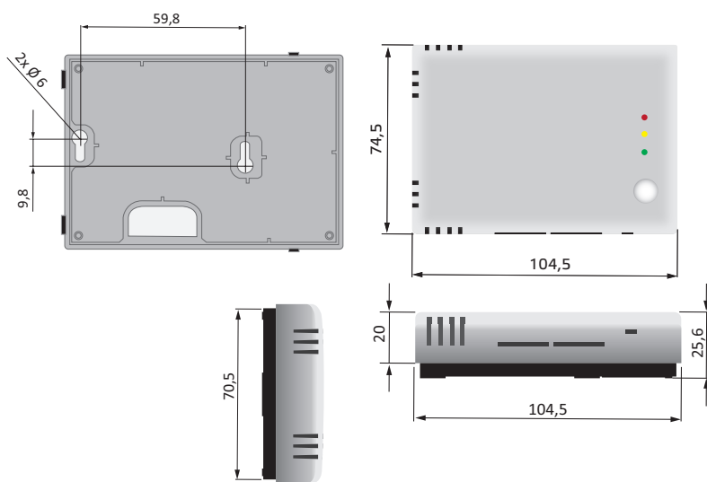
Мал. 2 Розміри для настінного монтажу
