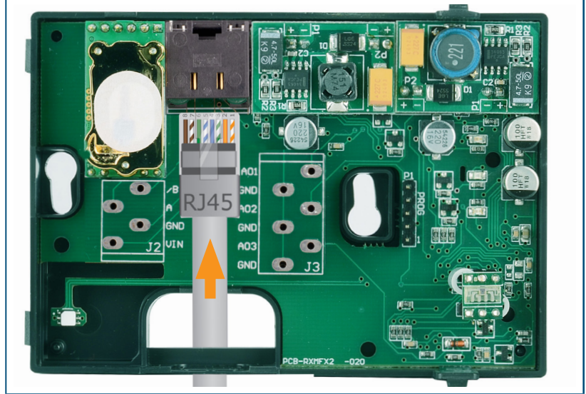
Мал. 4 Схема підключення
